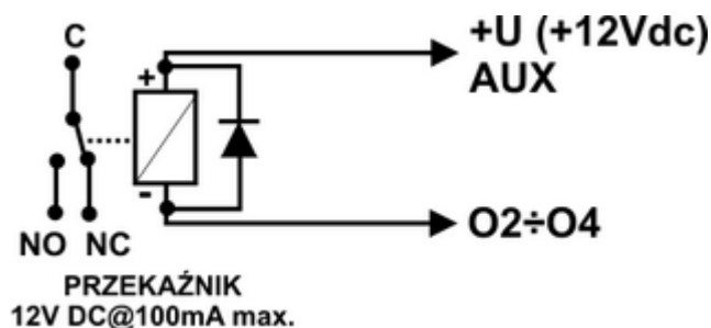
11 Podłączenie przekaźnika do wyjść O2 - O4.
