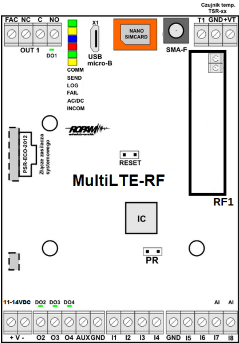
3 Widok MultiLTE-RF.
