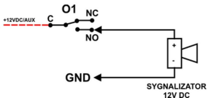
9 Przykład Podłączenia sygnalizatora (obciążenia) do wyjścia O1.
