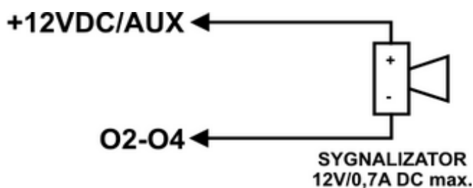
10 Przykład podłączenia sygnalizatora (obciążenia) do wyjść O2 - O4.
