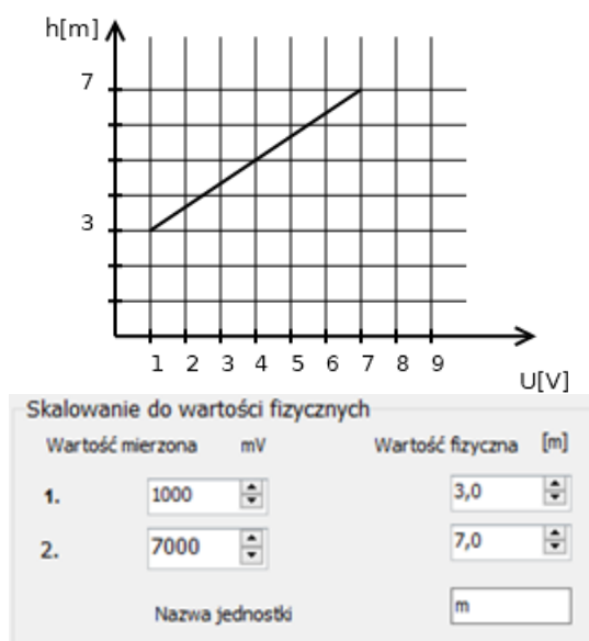
25 Zależność pomiędzy wielkością mierzoną a napięciem czujnika.
