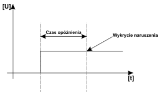
21 Opóźnienie zadziałania wejścia.
