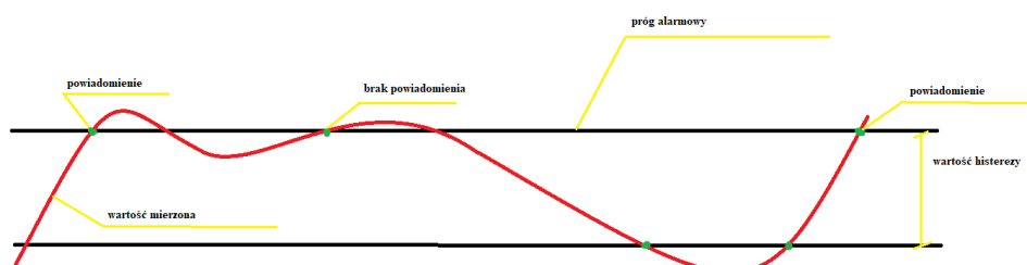
24 Graficzne przedstawienie histerezy.
