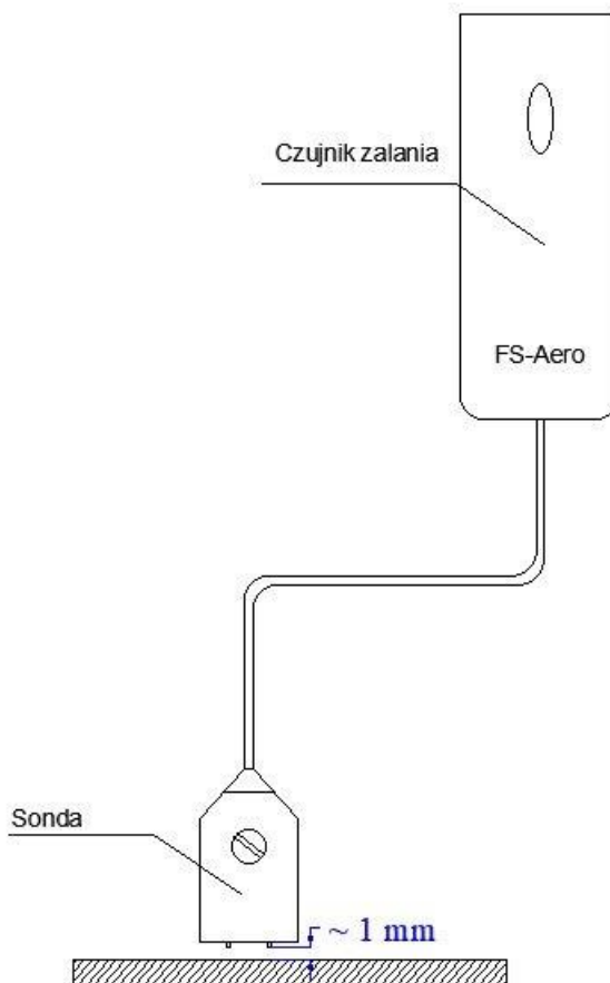
3 Sposób montażu sondy i czujnika.
