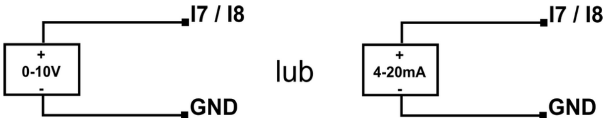
11 Podłączenie źródła napięciowego lub prądowego do wejść skonfigurowanych jako analogowe.
