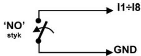
10 Wejście w konfiguracji NO
