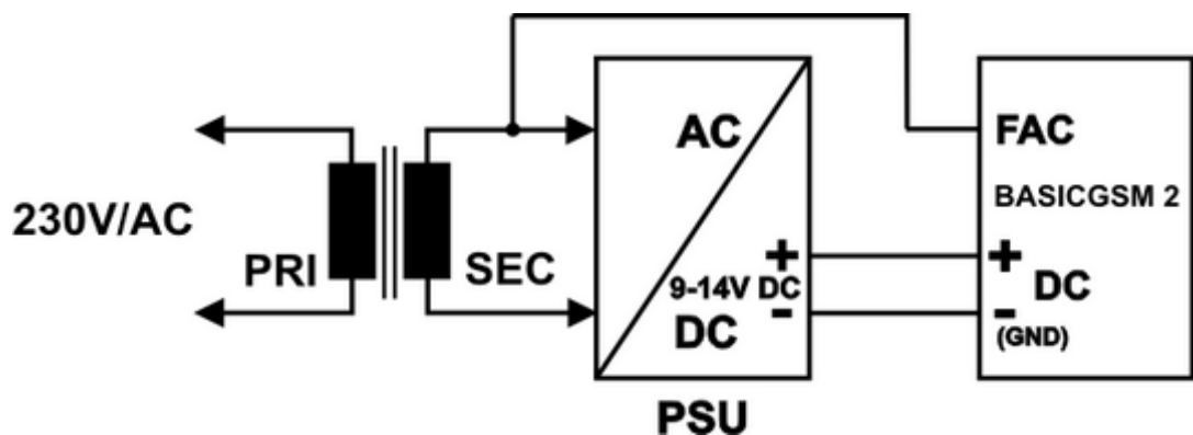
12 Podłączenie wejścia FAC do źródła napięcia AC.
