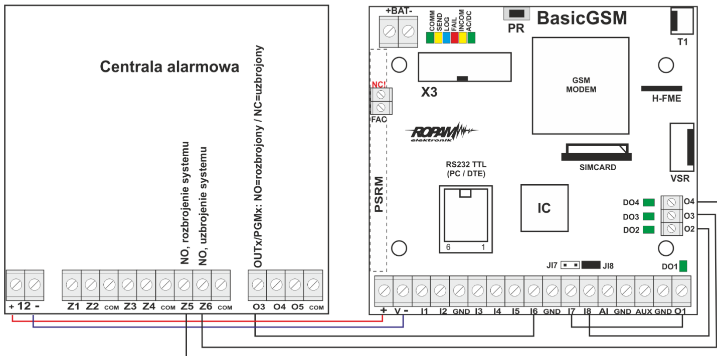
Rysunek 1 Przykładowy schemat podłączeń
